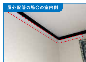
屋外配管の場合の室内側 屋内側の配線が内壁材の外側を通る場合があります。(赤点線部)
