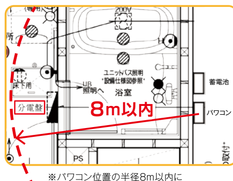
分電盤記載例
