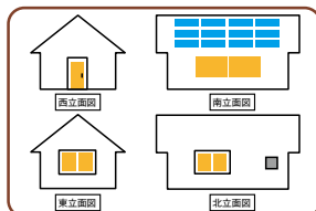
立面図
