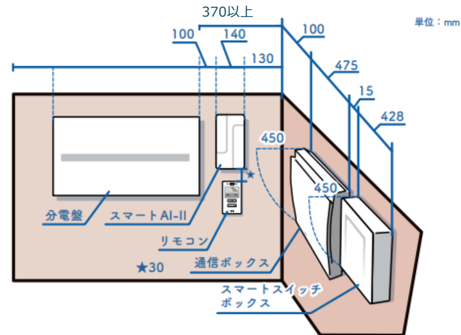
東京電力・中部電力・関西電力管轄での参考標準配置
