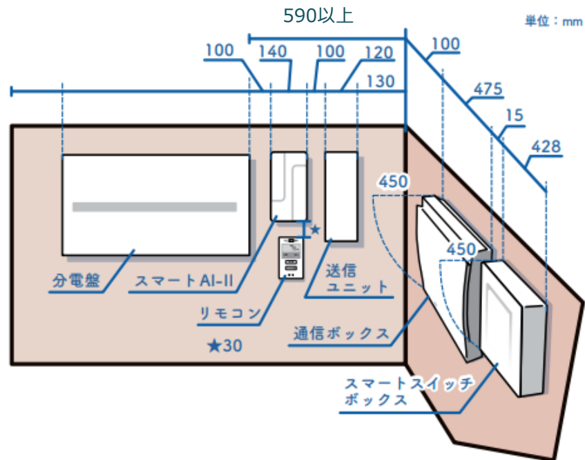
東北電力・中国電力・四国電力・九州電力管轄での参考標準配置
